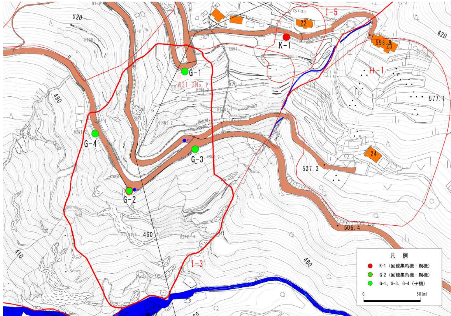
図 4 GNSS 動態計測対象地域の基準点及び計測点配置図
